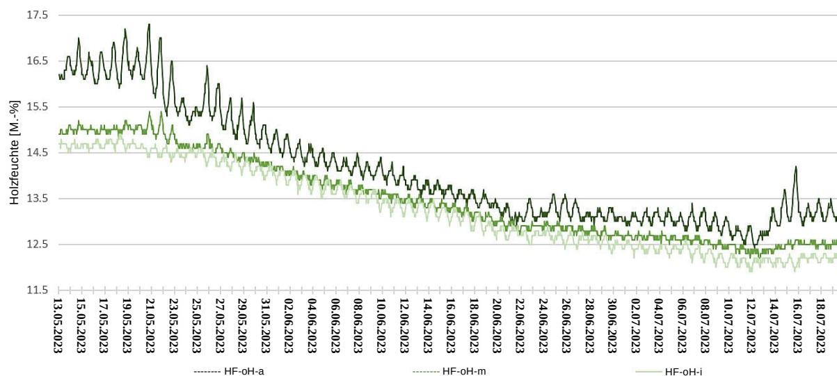
Abbildung 83: Holzfeuchteverlauf Selbstklimmer-Fassade nicht hinterlüftet ZR 2
