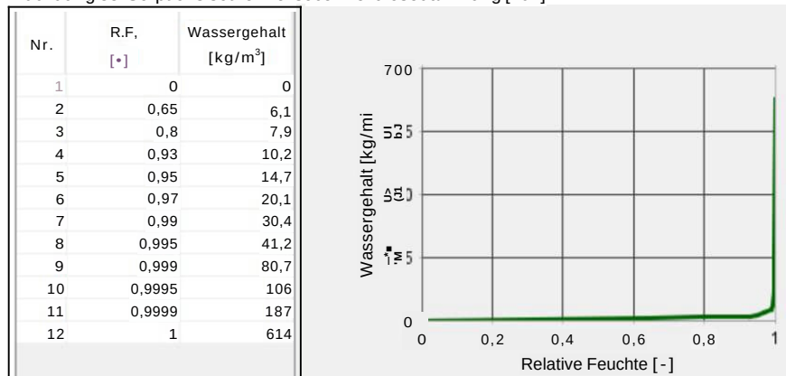
Abbildung 38: Sorptionsisotherme Isocell Zellulosedämmung [104]
