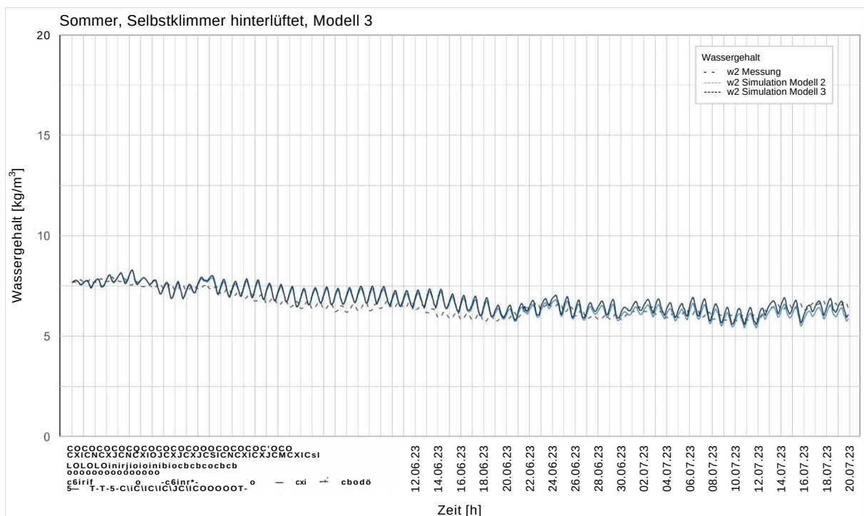
Abbildung A 52 Vergleich der Modelloptimierung in w2 von Modell 2 und Modell 3 der Fassade mH.
