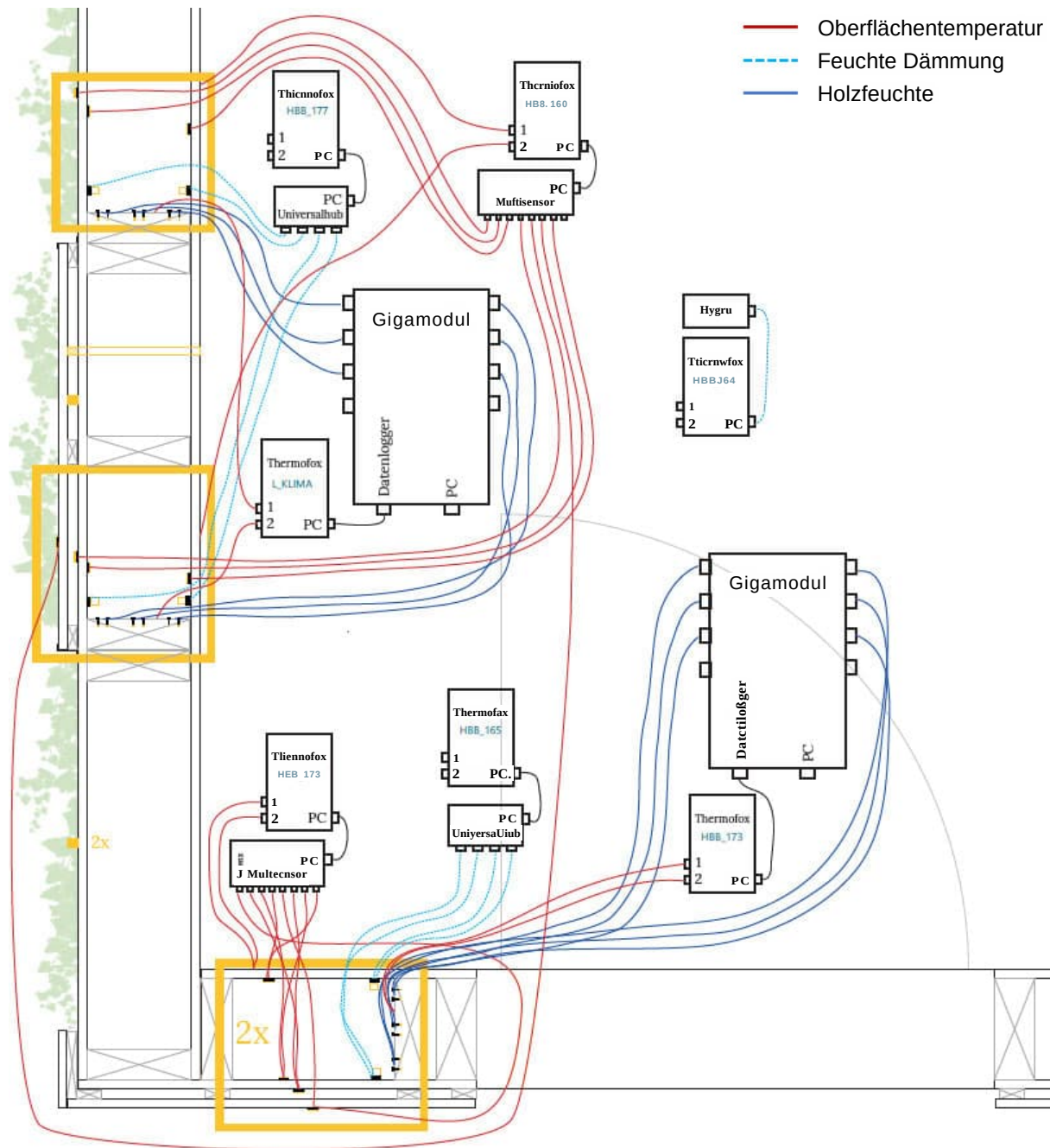
Abbildung 36: Ausschnitt der im Grundriss dargestellten Verkabelung der Messtechnik inklusive Beschriftung der Datenlogger (Thermofox Universal).
