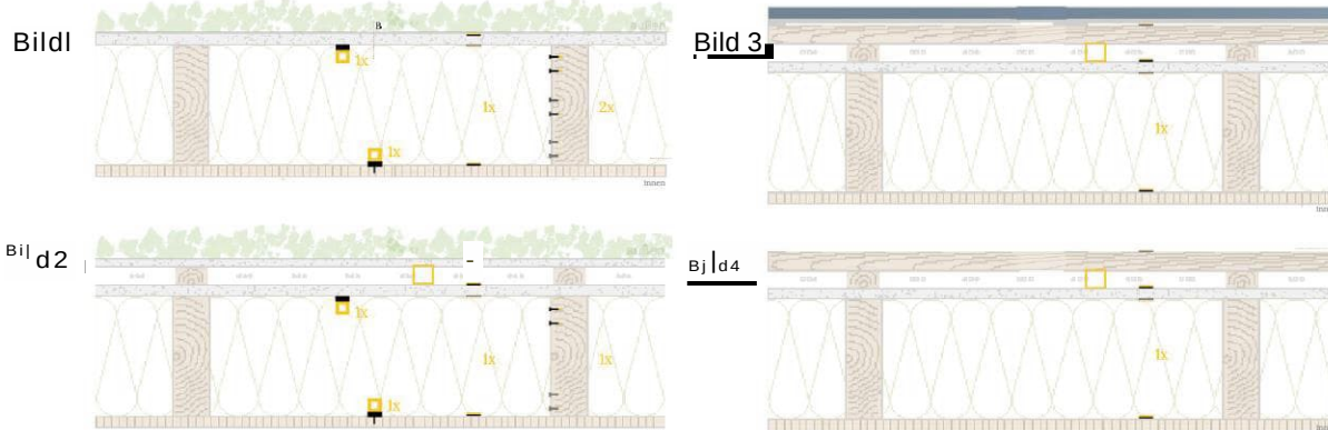
Abbildung 33: Positionierung der Sensoren in den Bauteilschichten; Bild 1: oH; Schnitt 2: mH; Schnitt 3: PV; Schnitt 4: Ref
