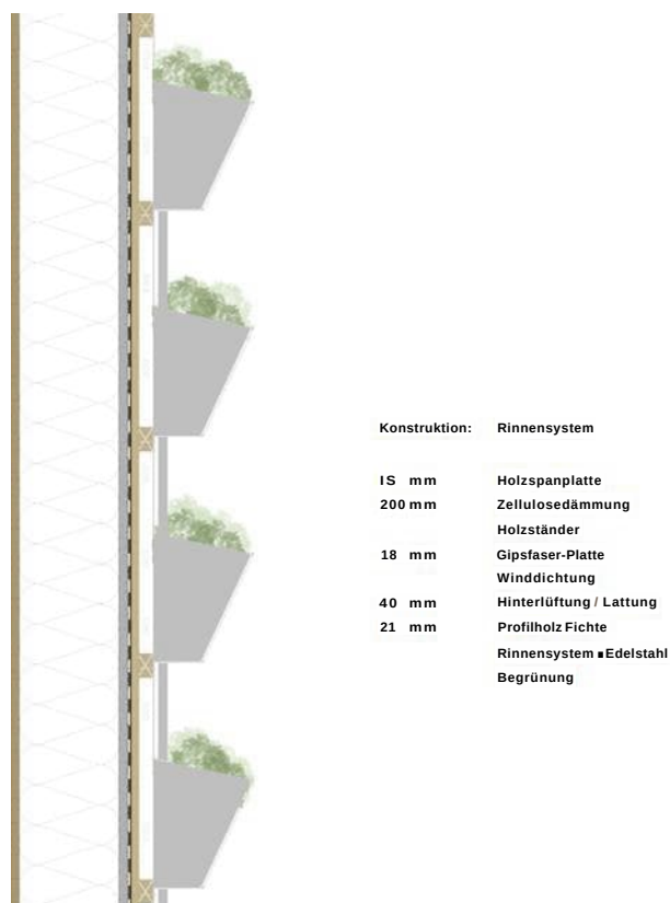
Abbildung 24 Visualisierung des Rinnensystems
