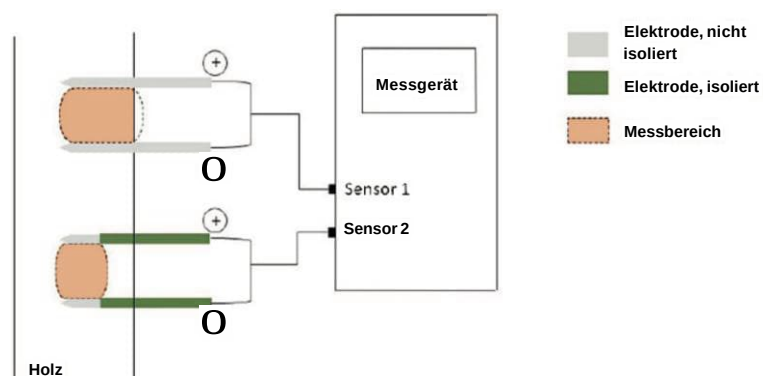
Abbildung 13 Elektrisches Widerstandsverfahren [42]
