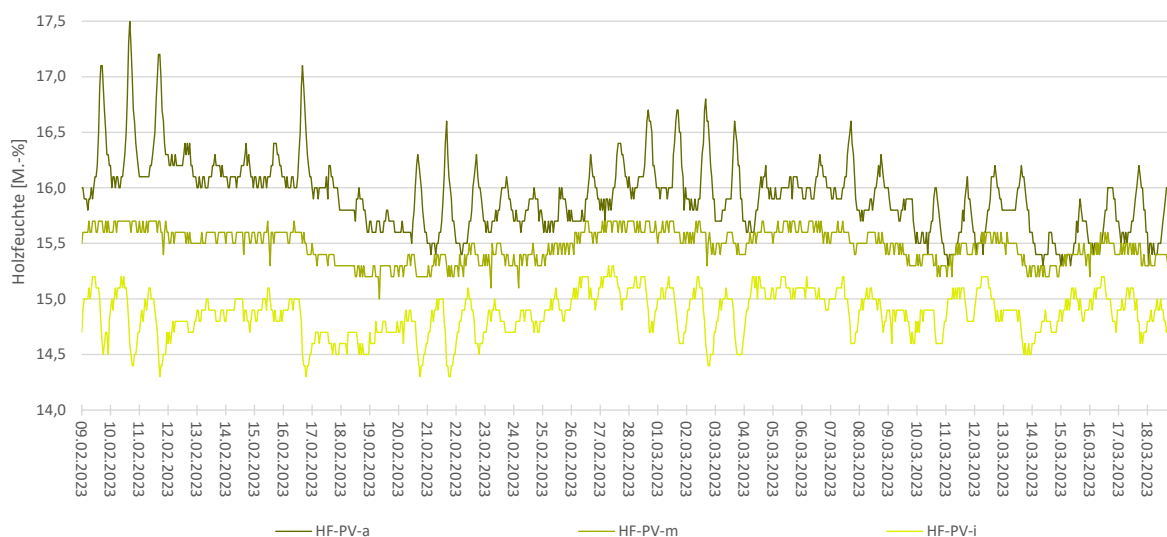
Abbildung 49: Holzfeuchtemessungen der Fassade mit PV
