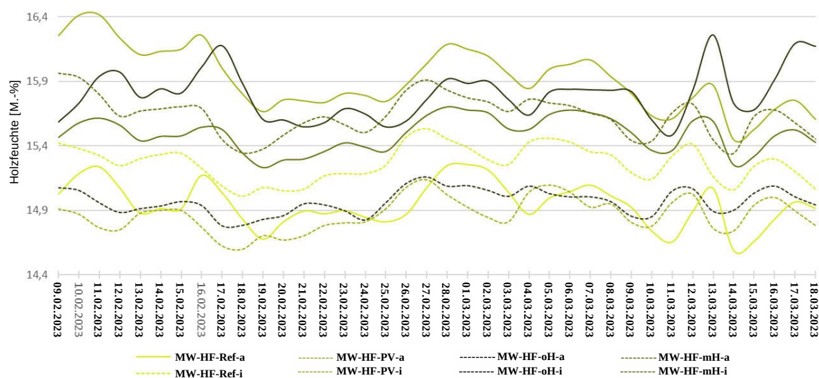
Abbildung 58: Holzfeuchteverlauf aller Fassadenpositionen a & i ZR 1
