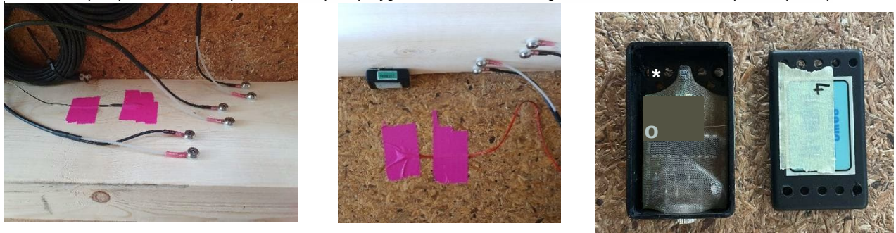
Abbildung 35: Eingebaute Messtechnik vor Befüllung mit Zellulosedämmung; Elektrisches Widerstandsverfahren zur Bestimmung der Holzfeuchte (links), Oberflächentemperatursensor (Mitte), Hygrosensor zur Bestimmung der Dämmfeuchte und -temperatur (rechts)
