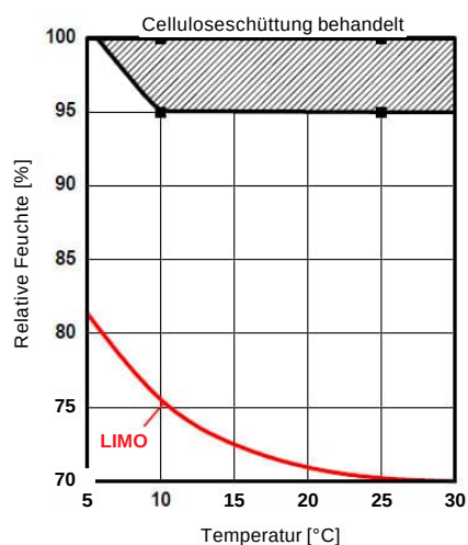
Abbildung 10: LIM-Kurve von Zellschüttung behandelt [34] (Hier ist der Versatz des Diagrammnullpunktes im Vergleich zu Abbildung 9 zu berücksichtigen.)
