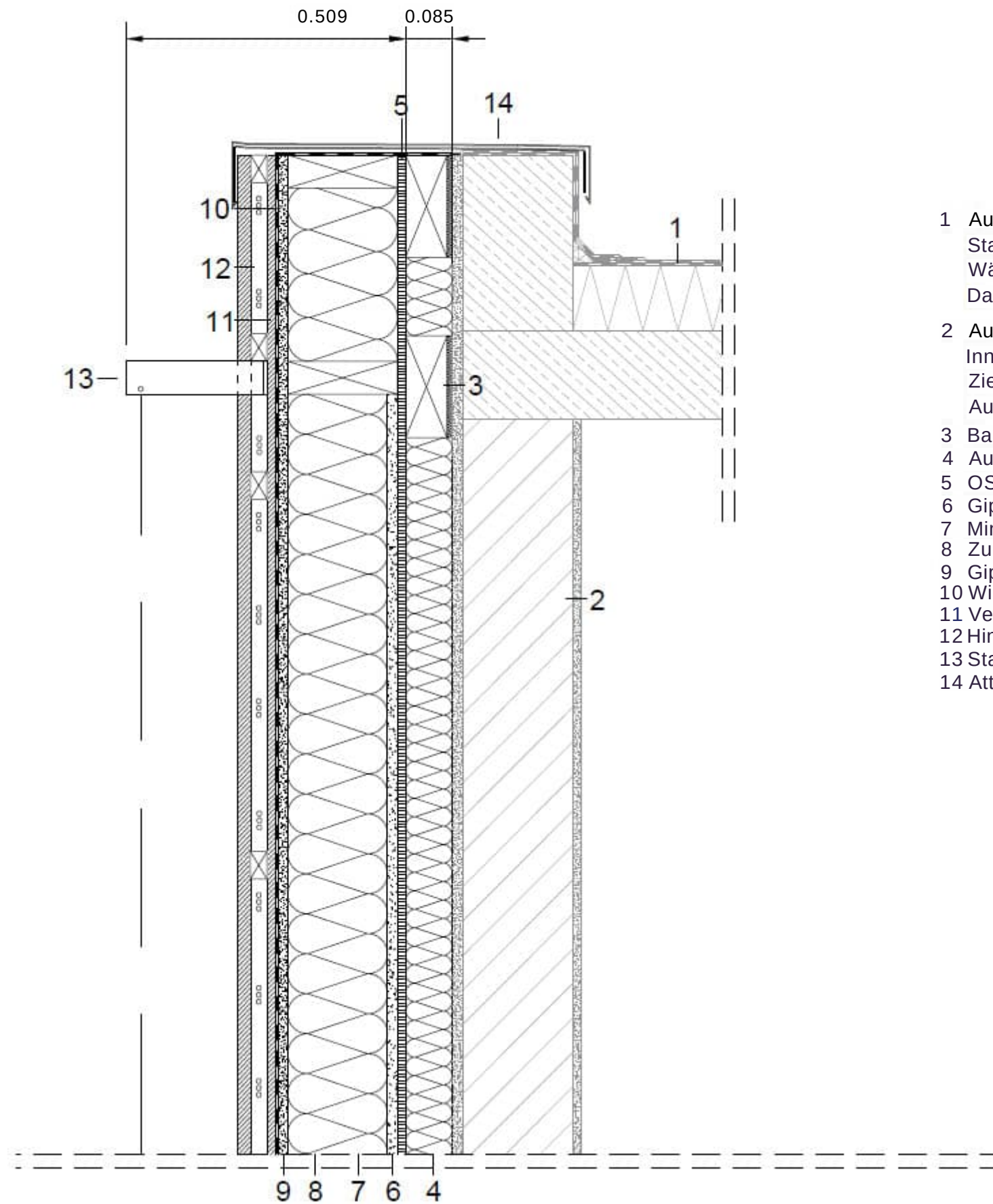
Abbildung A28 Detail - Trogsystem - Attikaelement - Schacht- Schnitt (maßstabslos)
