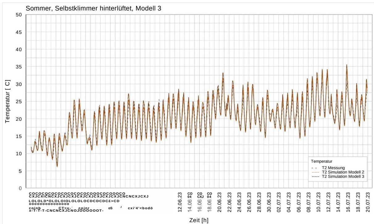
Abbildung A 51 Vergleich der Modelloptimierung in T2 von Modell 2 und Modell 3 der Fassade mH.
