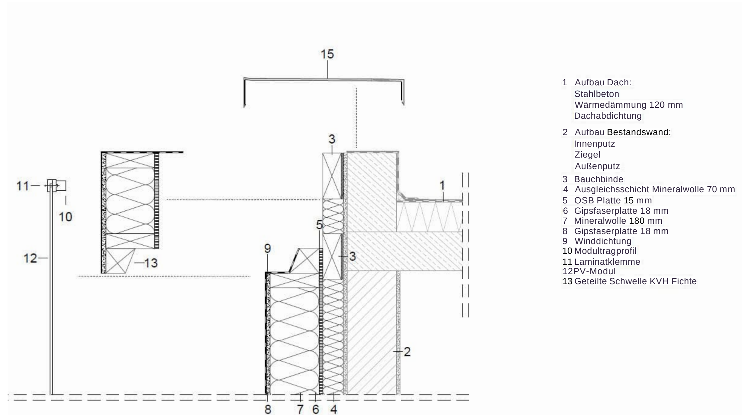
Abbildung A 10 Detail - Attikastoß - GES-Photovoltaik - Schnitt (maßstabslos)
