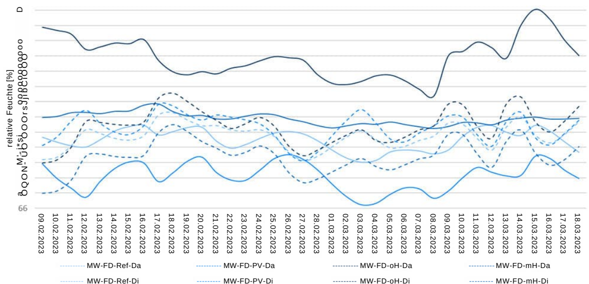
Abbildung 57: Verläufe der relativen Feuchte aller Fassaden in der Dämmebene ZR 1
