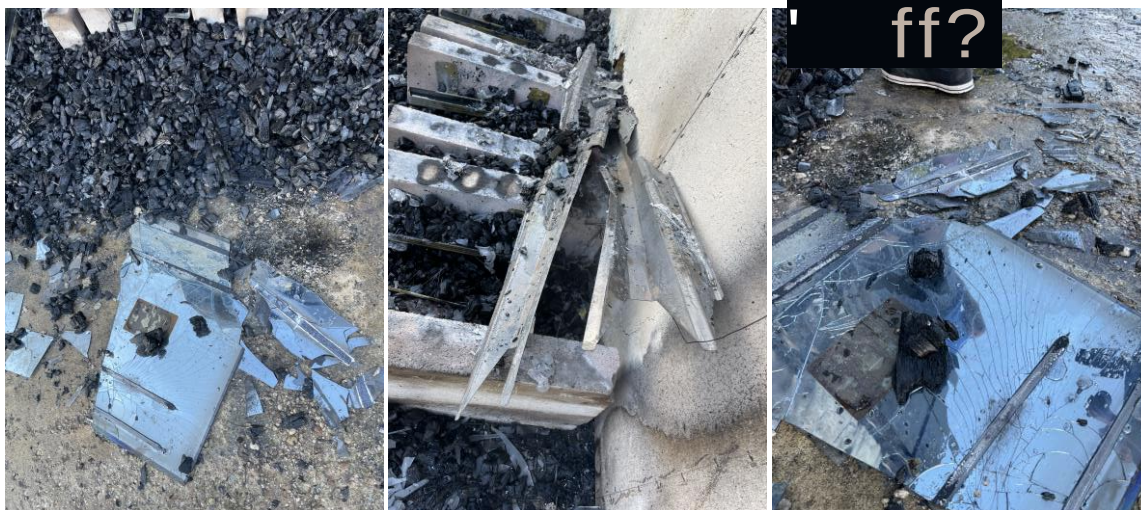
Abbildung 147: Bereich um den Prüfkörper nach dem Brandversuch
