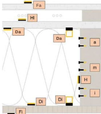
Abbildung 37: Abbildung der Sensorpositionen mit Benennung
