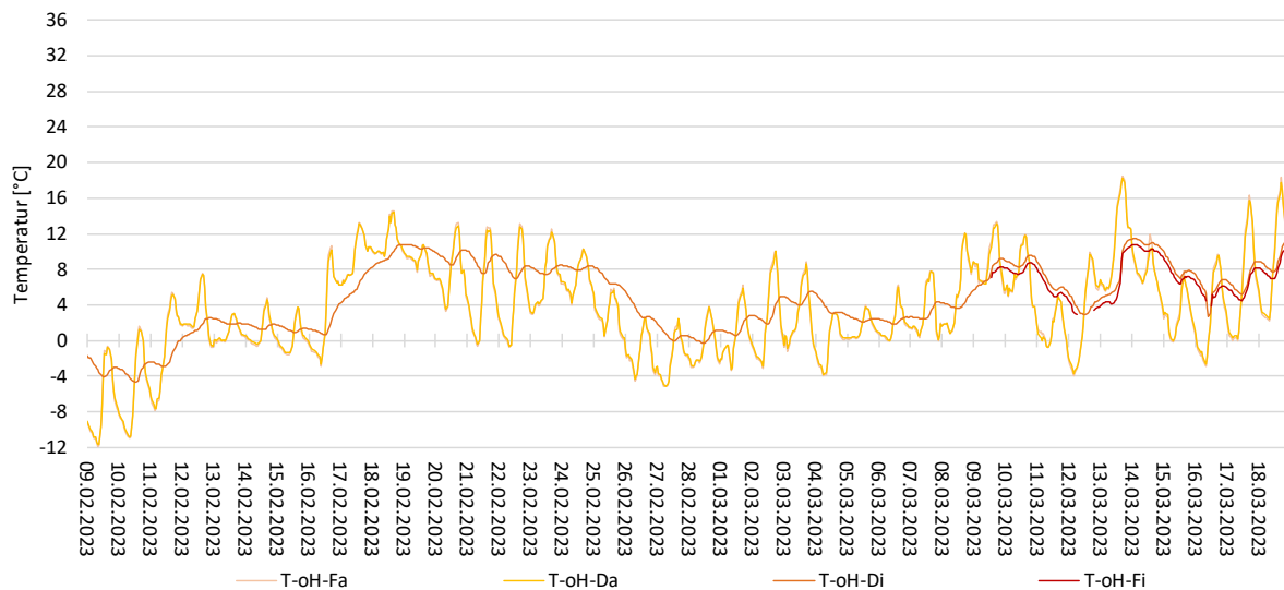
Abbildung 53: Messungen der Temperatur an der Fassade mit Begrünung ohne Hinterlüftung
