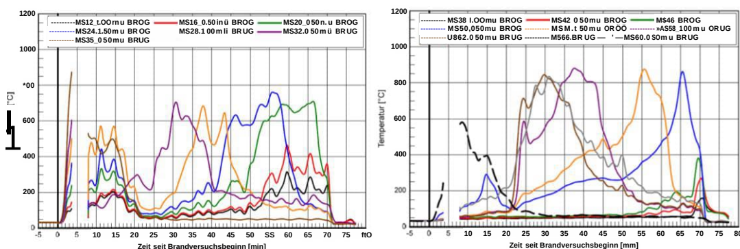
Abbildung 140: Temperaturverläufe in Achse 2 (Holzfassade), Ebene A vor der Fassade (links), Ebene B in der Hinterlüftung (rechts) ■
