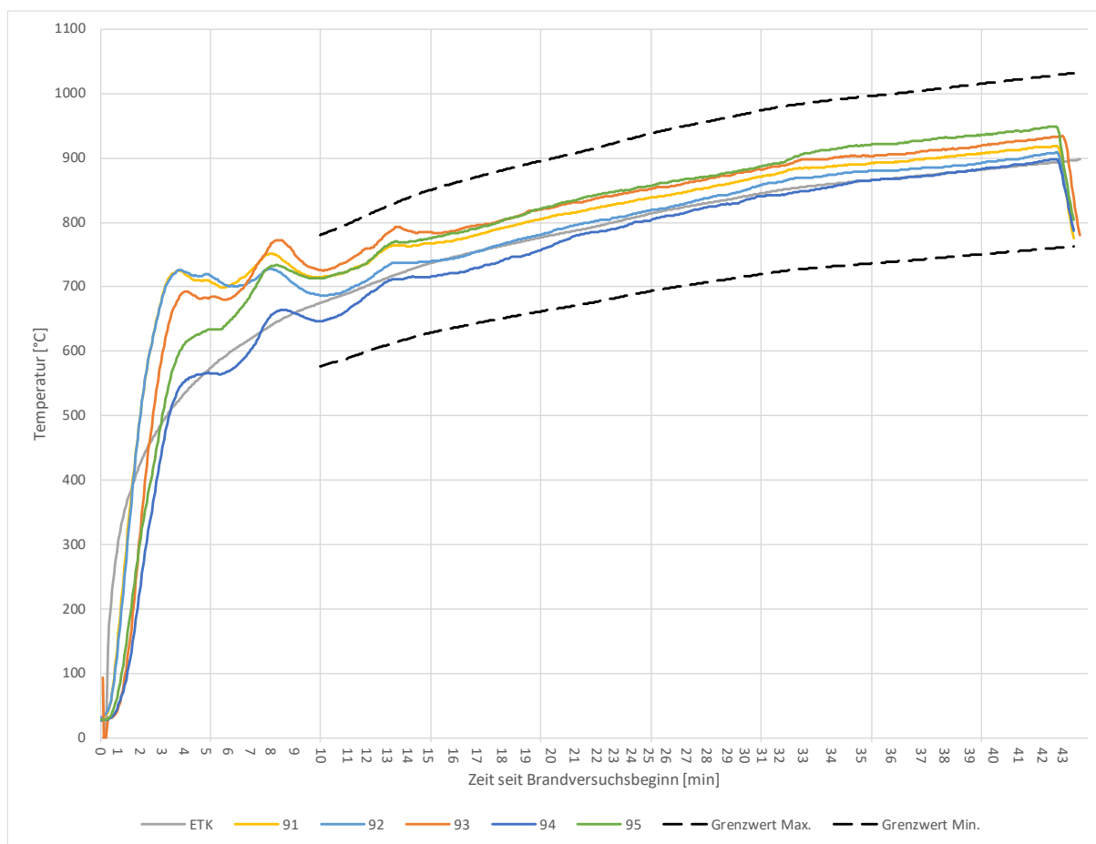
Abbildung 116: ETK und Brandraumtemperatur
