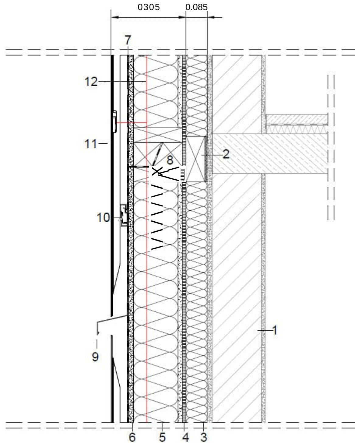
Abbildung A5 Detail - Eckverbindung - AVANCIS Skala - Grundriss (maßstabslos)
