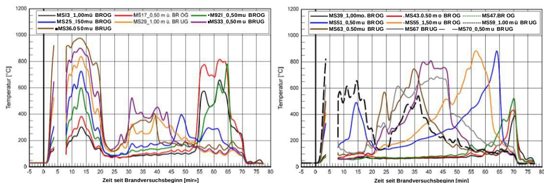
Abbildung 141: Temperaturverläufe in Achse 3 (Photovoltaikfassade), Ebene A vor der Fassade (links), Ebene B in der Hinterlüftung (rechts)
