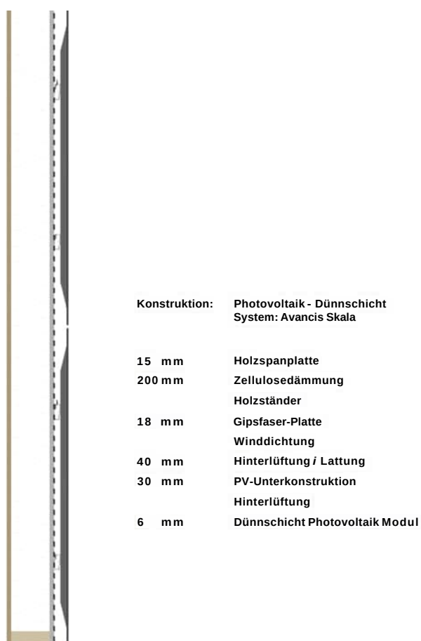
Abbildung 26 Visualisierung Photovoltaik AVANCIS-Skala-System
