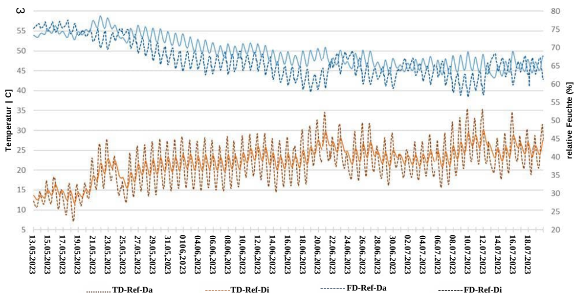
Abbildung 66: Verläufe der relativen Feuchte und Temperatur in der Dämmebene Referenzfassade ZR 2
