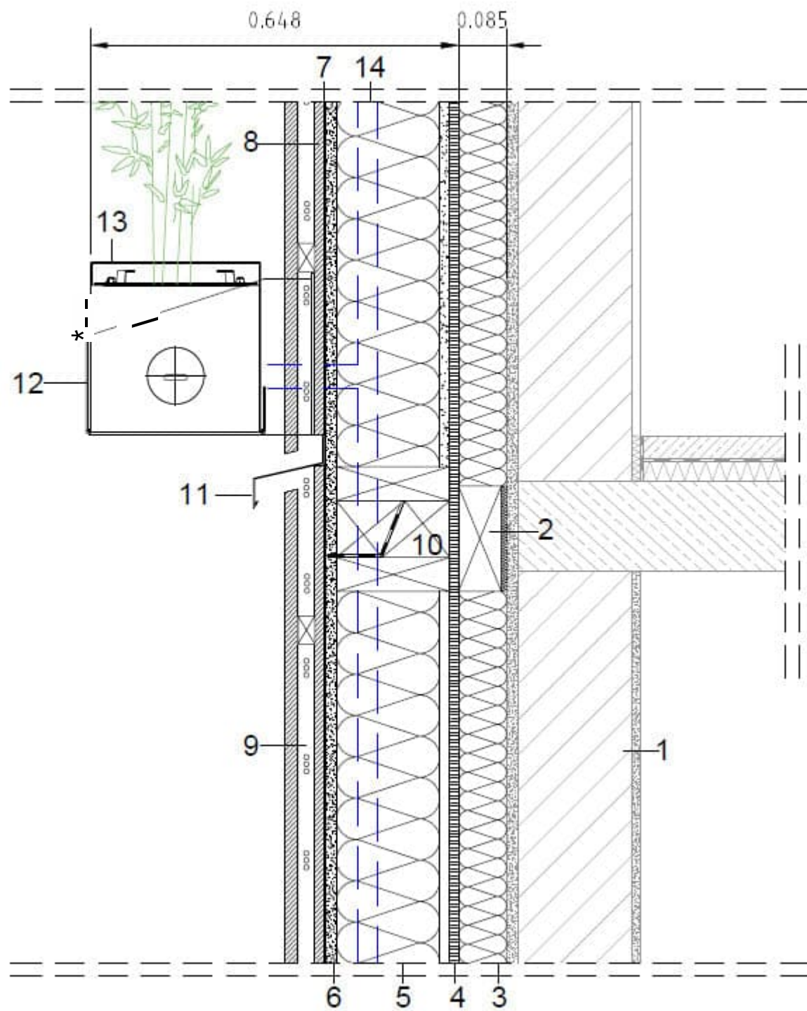
Abbildung A30 Detail - Trogsystem - Elementstoß - Schacht - Schnitt (maßstabslos)
