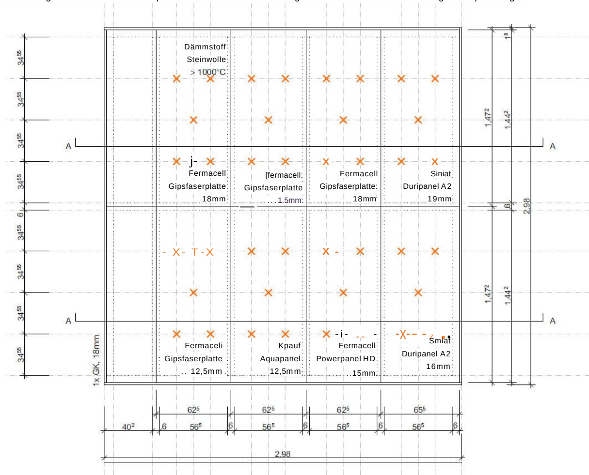
Abbildung 111: Ansicht des Prüfkörpers mit vertikaler Positionierung der Thermoelemente innenseitig der Beplankungen
