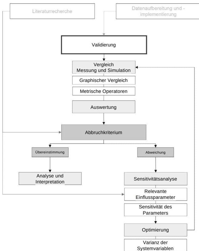
Abbildung 99 Validierungsmethodik
