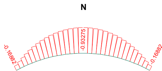
Bild 7.2-9: Querschnitt in Schalenmitte, Normalkraft [kN/Roststab] bei einer Last von p=11,23 \text{ kN/m}^2 .
