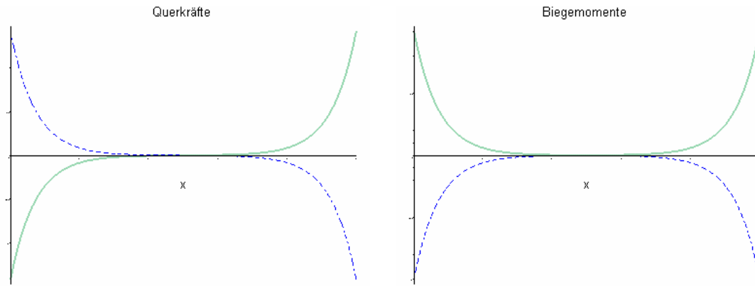
Bild 4.5-3: Lastfall „gegenseitige Randmomente“: Beispielhafter, qualitativer Verlauf der Schnittgrößen (Ebene A gestrichelt, Ebene B durchgezogene Kurve)
