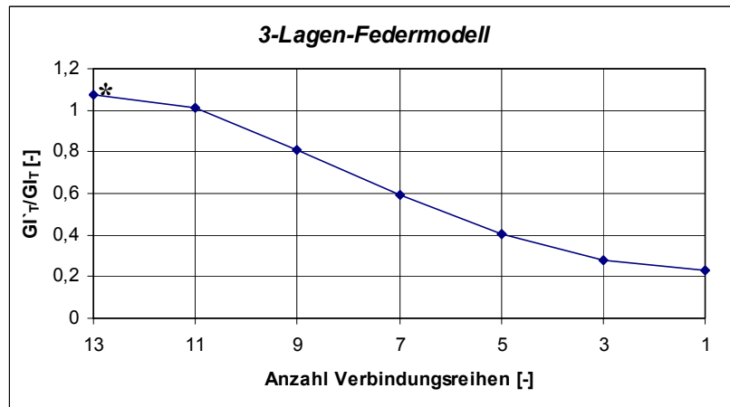
Bild 6.4-3: Dreiteiliger Verbundquerschnitt: Verhältnis von effektiver Torsionssteifigkeit GI_T' zur Torsionssteifigkeit GI_T bei starrem Verbund in Abhängigkeit von der Anzahl der Verbindungsreihen (Reduzierung von aussen zur Querschnittsmitte).
