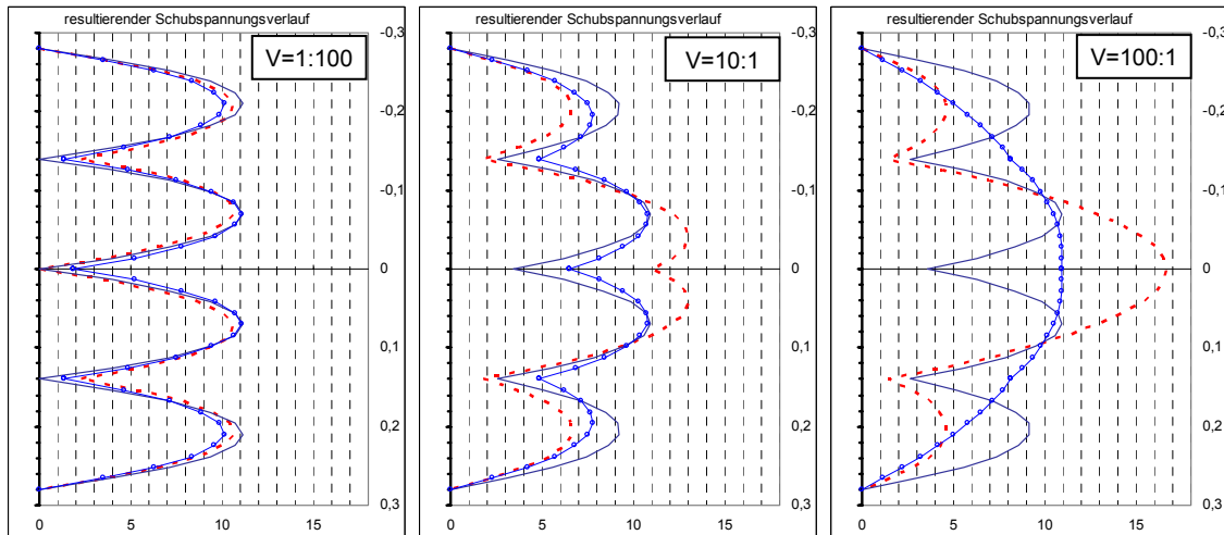
Bild 5.5-23: Schubspannungsverläufe (Auflagerbereich) am verdübelten Balken für V=c_{23}/c_{12}=\{1:100; 10:1; 100:1\} (bei einer Last von P=1000 kN)
