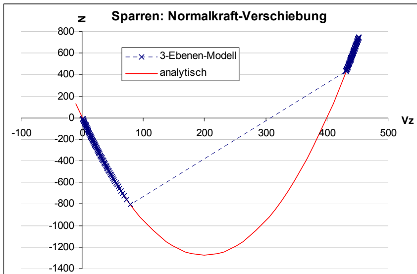
Bild 4.6-18: Normalkraft-Verschiebungs-Kurve Sparrenkonstruktion; Ergebnisse Iteration Drei-Ebenen-Modell mit x gekennzeichnet
