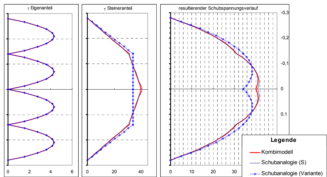
Bild 5.5-6: In ihre Anteile aufgegliederte Schubspannungsverläufe am Verbundquerschnitt des Beispielträgers für verschiedene Fugensteifigkeiten [\text{MPa} \cdot 10^3] (bei p_0=1\text{kN} ). Vergleich der Lösung gemäß der Schubanalogie mit dem Referenzwert ( \gamma -Verfahren, gestrichelt).
