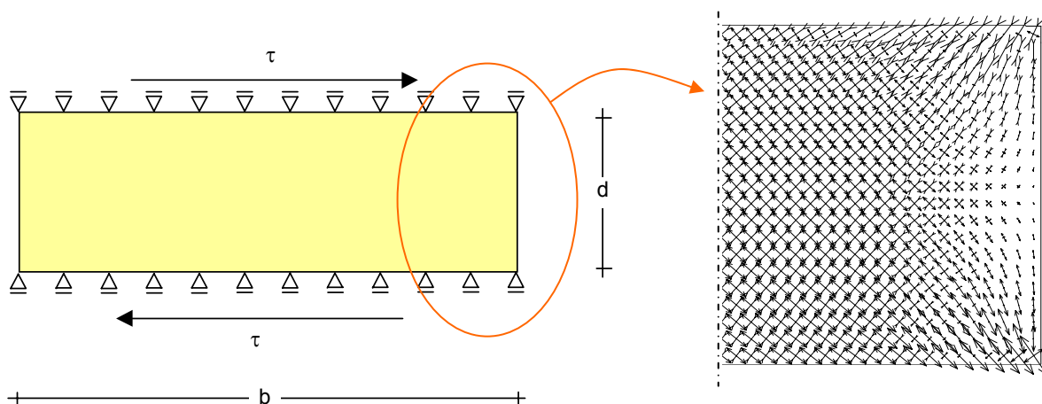
Bild 6.2-5: Rechnerische Untersuchung am „Schubblockmodell“; links System mit Belastung, rechts vektorielle Darstellung der Hauptspannungen am rechten Rand; \leftrightarrow Zug, \rightarrow Druck.
