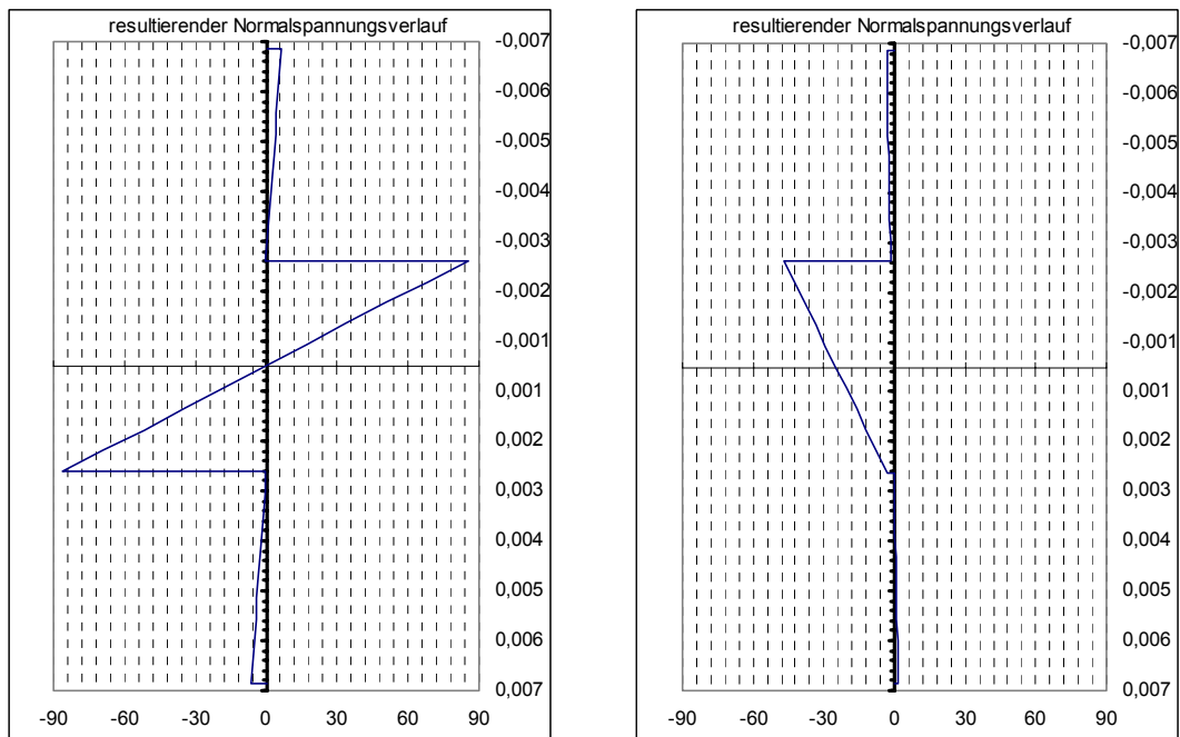
Bild 7.2-30: Normalspannungen [MPa] in Längsrichtung. Links: im Bereich der Querscheibe; rechts: in Schalenmitte.
