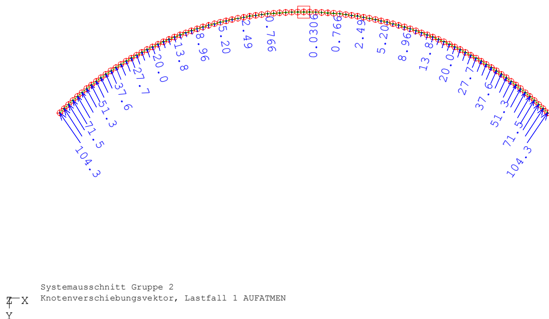
Bild 7.1-8: Programmausdruck: Verformungsfigur und Knotenverschiebungen [mm] des verschraubten Bogens, Lastfall „Aufatmen“, Darstellung der Ebene B=Gruppe 2
