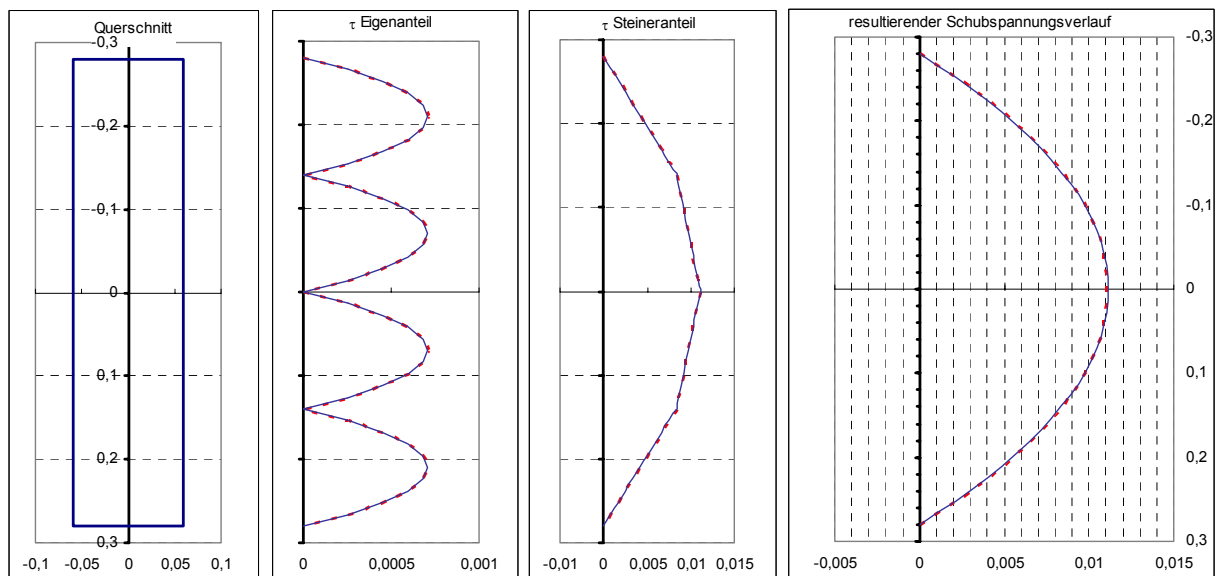
Bild 5.5-13: Vergleich der Ergebnisse für die Schubspannungsverteilung am verdübelten Balken im Auflagerbereich. Gestrichelt: Werte gemäß dem kombinierten Modell. Werte in [MPa] pro [kN] Last.
