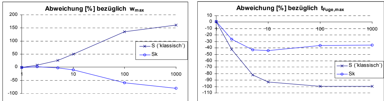
Bild 5.5-32: Abweichung [%] (Ordinate) der Schubanalogie zum Fachwerkmodell in Abhängigkeit vom Verhältnis der Fugensteifigkeiten ( V , Abszisse, logarithmisch skaliert) in Bezug auf die maximalen Schub- und Normalspannungen.
