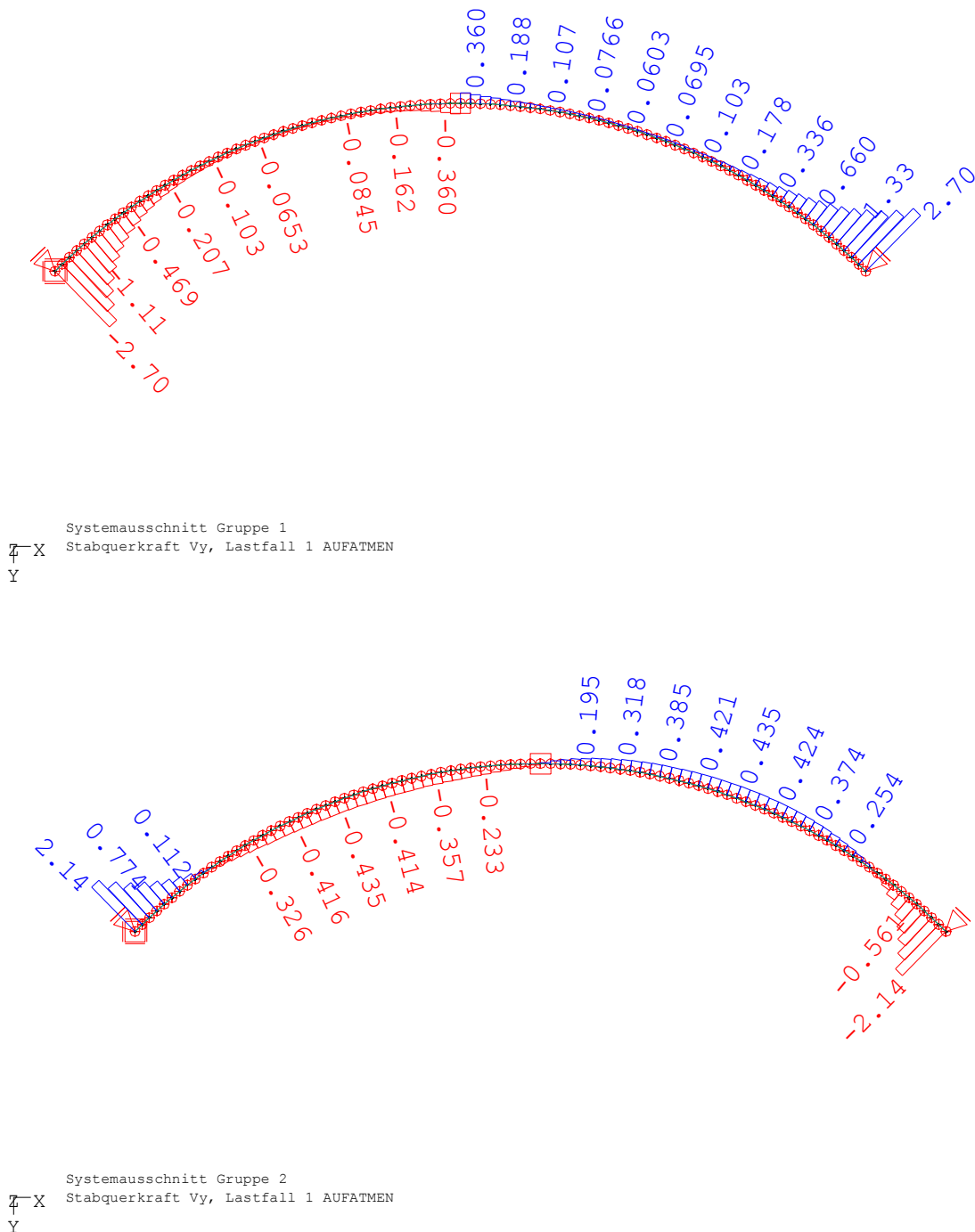
Bild 7.1-9: Programmausdruck: Querkraftverlauf [kN] am ideellen System, Lastfall „Aufatmen“; Gruppe 1 ≡ Ebene A, Gruppe 2 ≡ Ebene B
