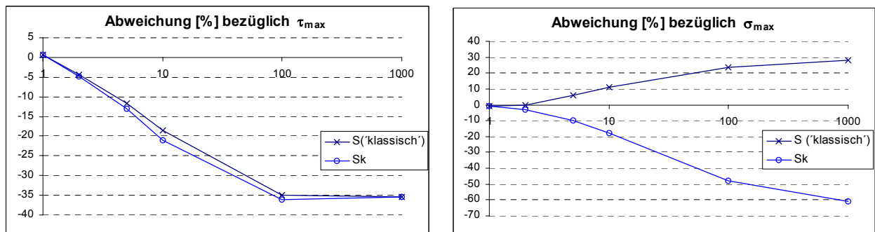
Bild 5.5-33: Abweichung [%] (Ordinate) der Schubanalogie zum Fachwerkmodell in Abhängigkeit vom Verhältnis der Fugensteifigkeiten ( V , Abszisse, logarithmisch skaliert) in Bezug auf die maximale Durchbiegung w und den maximalen Schubfluss in der Verbundfuge
