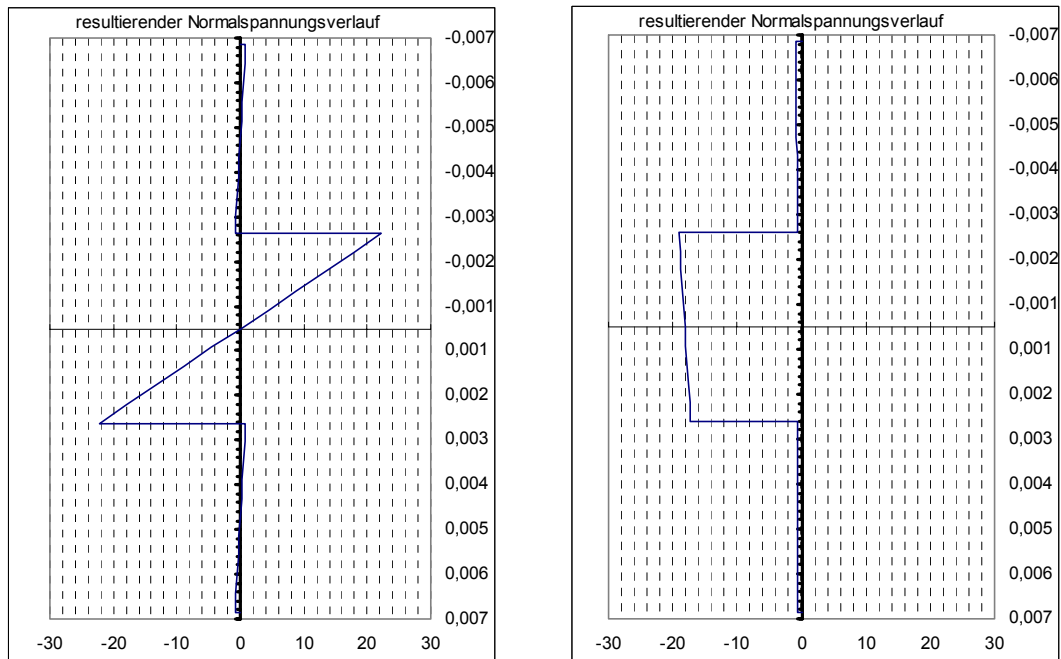
Bild 7.2-15: Normalspannungen [MPa] in Längsrichtung. Links: im Bereich der Querscheibe; rechts: in Schalenmitte.
