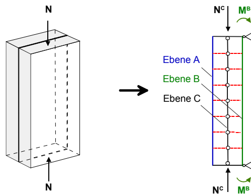
Bild 4.7-1: Einseitig belasteter Verbundquerschnitt, Transformation zum ideellen Rechensystem
