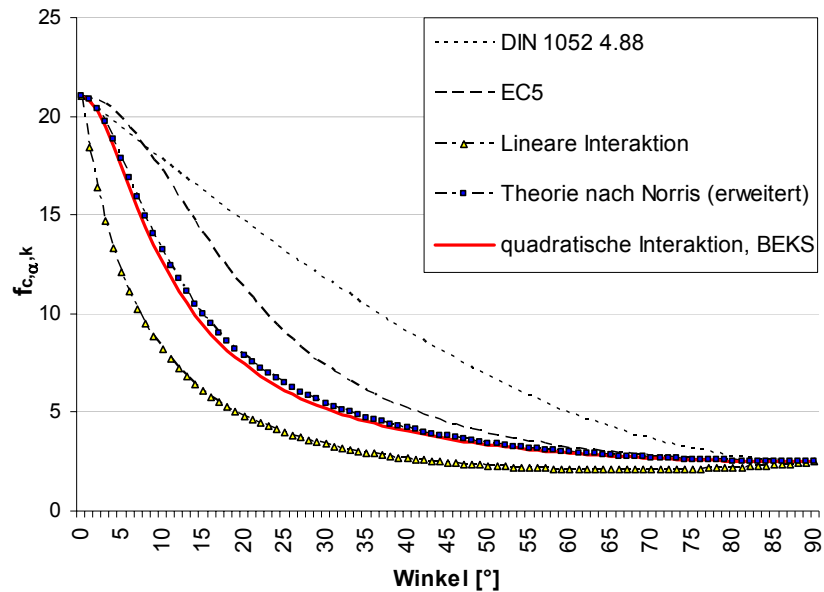
Bild 6.3-6: Vergleich der Ansätze für den Anwendungsfall „Druck unter einem Winkel zur Faser“. Bestimmung der charakteristischen Festigkeit f_{c,\alpha,k} auf Basis der charakteristischen Festigkeiten für NH CD24 nach [N4] ( f_{c,0,k}=21 MPa, f_{c,90,k}=2,2 MPa, f_{v,k}=2,7 MPa).
