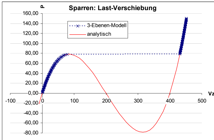
Bild 4.6-17: Last-Verschiebungs-Kurve Sparrenkonstruktion; Ergebnisse Iteration Drei-Ebenen-Modell mit x gekennzeichnet
