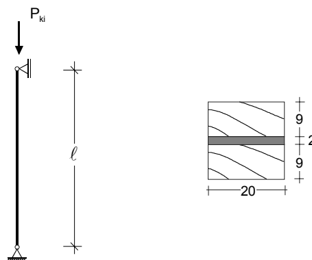
Bild 4.6-3: Links: System Testbeispiel; rechts: zugehöriger Stabquerschnitt.
