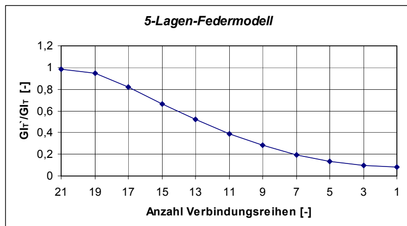
Bild 6.4-5: Fünfteiliger Verbundquerschnitt: Verhältnis von effektiver Torsionssteifigkeit GI_T' zur Torsionssteifigkeit GI_T bei starrem Verbund in Abhängigkeit von der Anzahl der Verbindungsreihen (Reduzierung von außen zur Querschnittsmitte).
