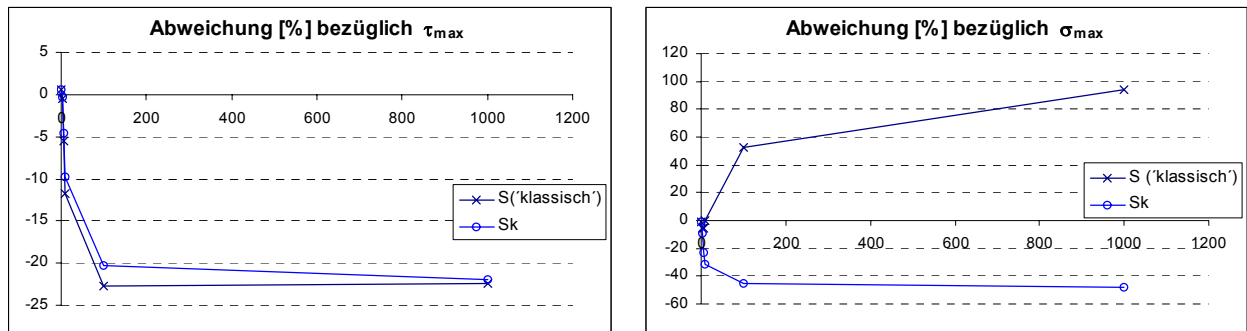
Bild 5.5-29: Abweichung [%] (Ordinate) der Schubanalogie zum Fachwerkmodell in Abhängigkeit vom Verhältnis der Fugensteifigkeiten ( V , Abszisse, logarithmisch skaliert) in Bezug auf die maximale Durchbiegung w und den maximalen Schubfluss in der Verbundfuge
