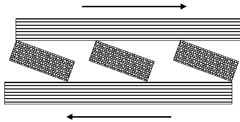
Bild 6.2-4: Gedankenmodell zur Veranschaulichung des Entstehens von Normalspannungen in den Querlagen infolge einer Schubbelastung
