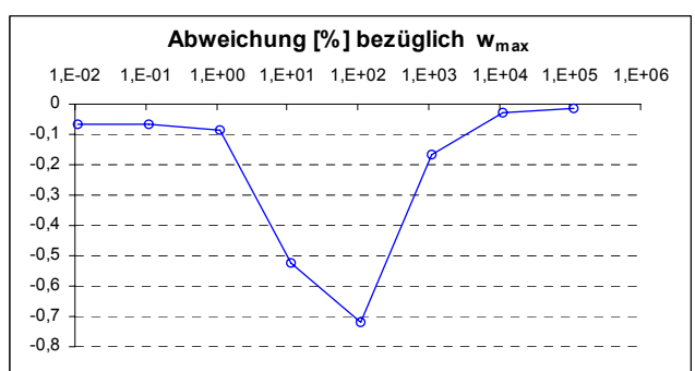
Bild 5.5-17: Vergleich der Maximalwerte für den Schubfluss in den Verbundfugen [MPa] und die Durchbiegung w [m] (oben); darunter: Abweichungen bezogen auf den Referenzwert [%]. Darstellung in Abhängigkeit von der Fugensteifigkeit (Abszisse, logarithmisch skaliert)
