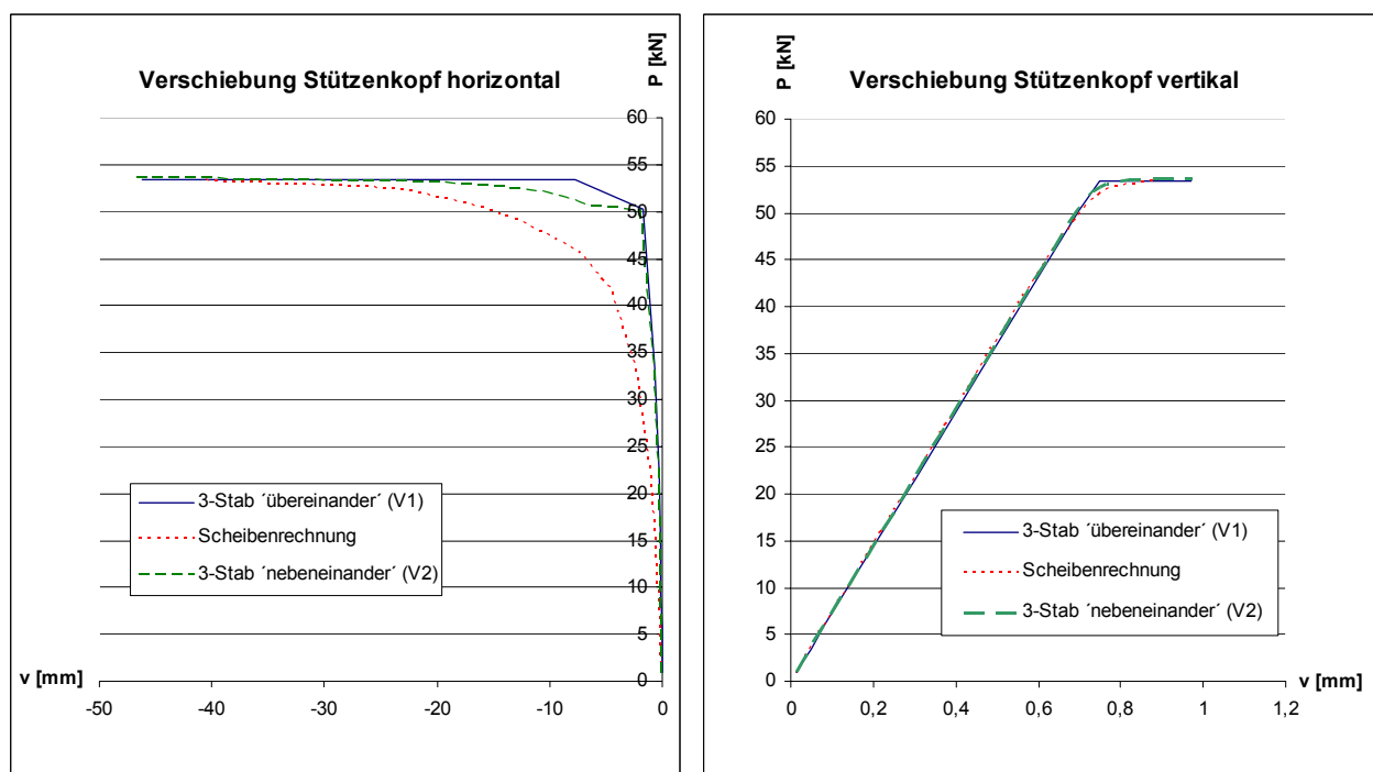
Bild 4.6-8: Vergleich der Last Verschiebungskurven aus Scheibenrechnung und nach Schubanalogie (Varianten V1 und V2) für den einhäufigen Rahmen
