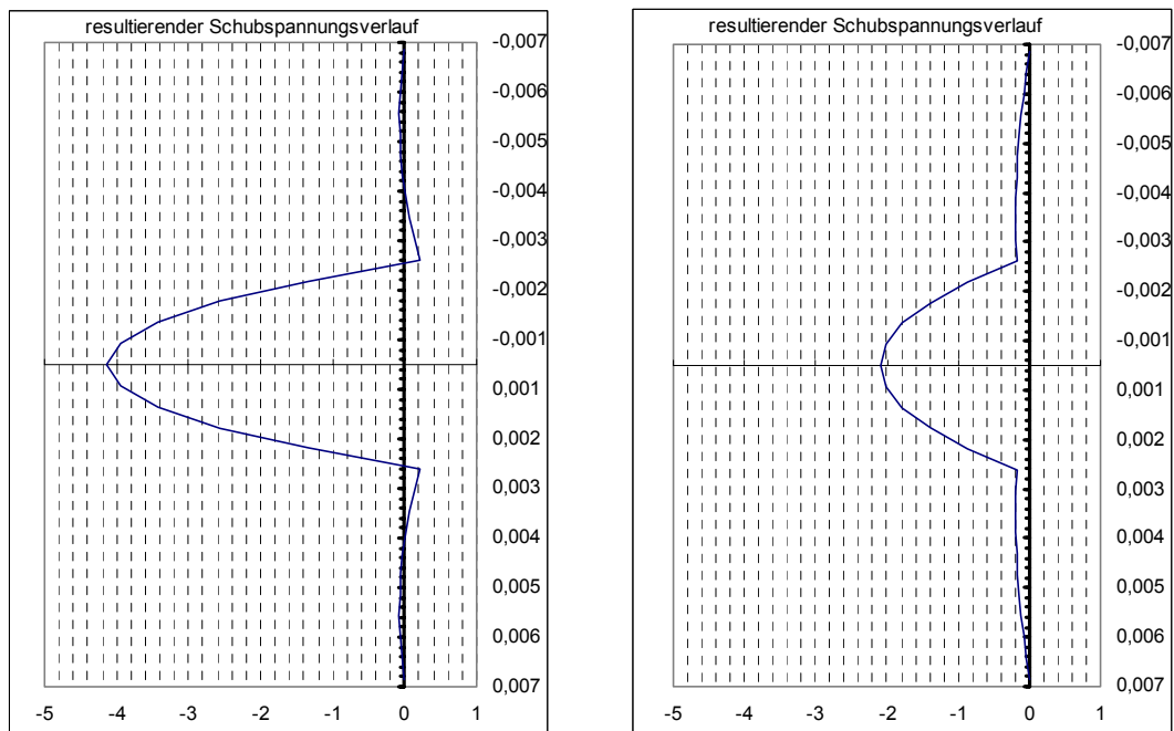
Bild 7.2-31: Schubspannungen [MPa] am Schnitt quer zur Längsrichtung. Links: Schnitt 2 cm vor der der Endquerscheibe; rechts: Schnitt ca. 6 cm vor der Endquerscheibe.
