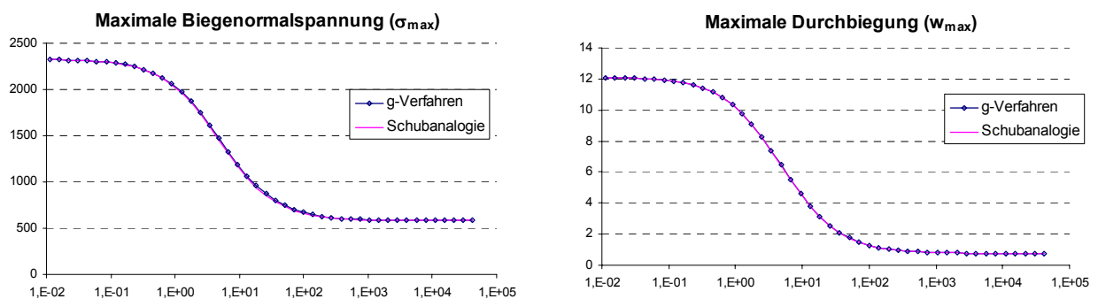
Bild 5.5-2: Vergleich der maximalen Biege­normalspannung [MPa·10 3 ] und der maximalen Durchbiegung [mm] (bei p 0 =1kN). Darstellung in Abhängigkeit von der Fugensteifigkeit [MPa] (Abszisse, logarithmisch skaliert).
