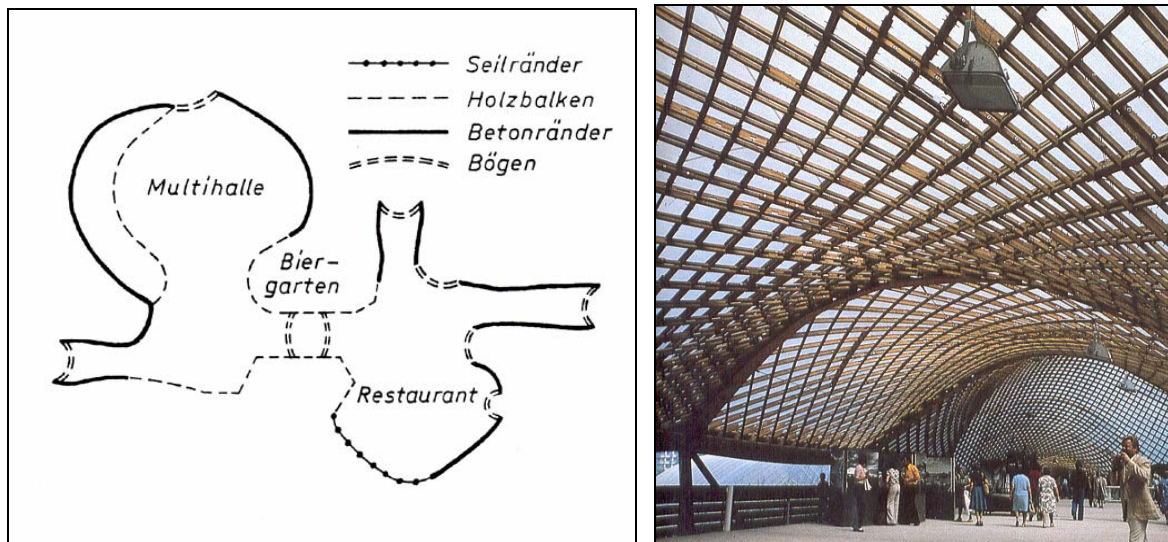
Bild 3.2-11: Multihalle Mannheim: links: Grundriss und Randträgertypen, rechts: Innenansicht. (Quellen: [98] bzw. [34])
