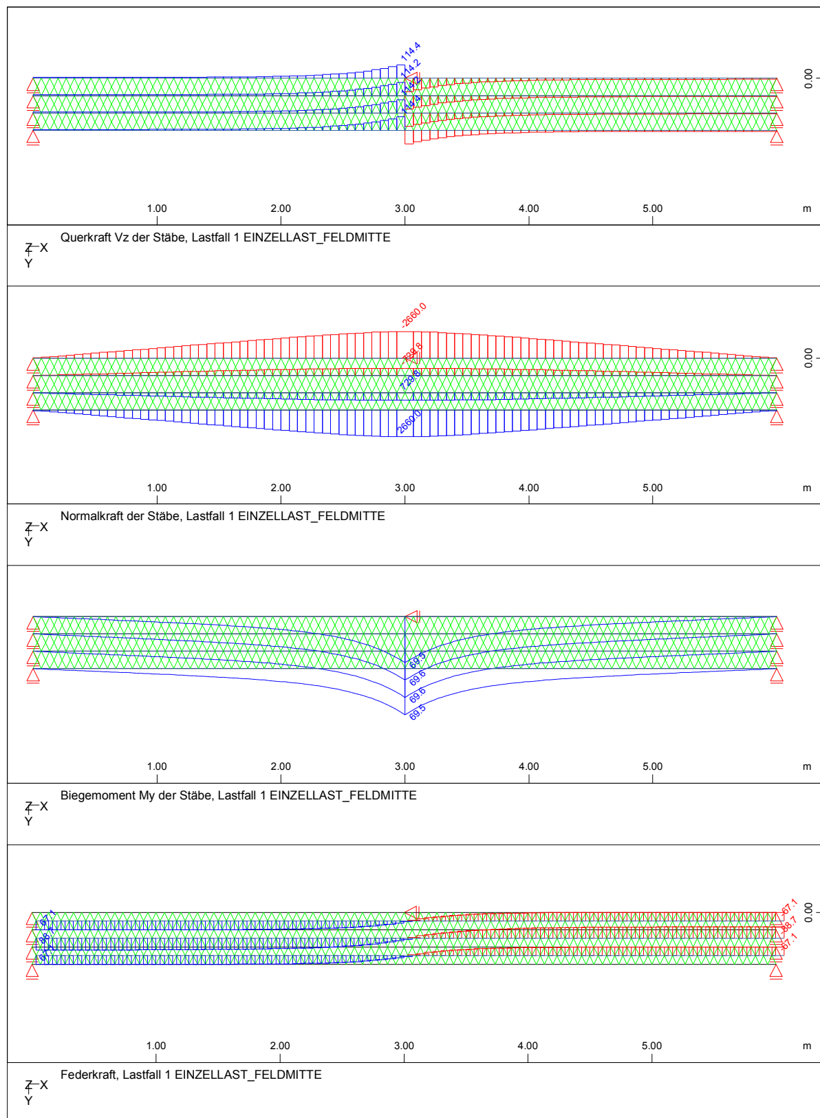
Bild 5.5-14: Programmausdruck der Ergebnisse gemäß dem kombinierten Modell für den vierteiligen verdübelten Balken bei einer Last von P=1000 \text{ kN}
