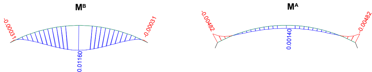
Bild 7.2-23: Querschnitt in Schalenmitte, ideelle Biegemomente [\text{kNm/Roststab}] bei einer Last von p=3,81 \text{ kN/m}^2 .
