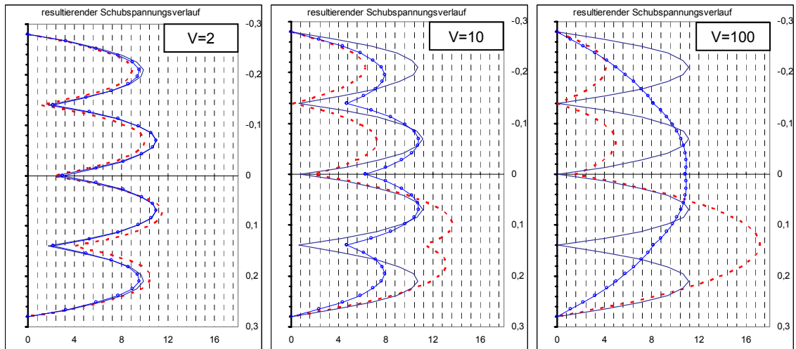
Bild 5.5-31: Schubspannungsverläufe (Auflagerbereich) am verdübelten Balken für V=\{2; 10; 100\} (bei einer Last von P=1000 \text{ kN} )
