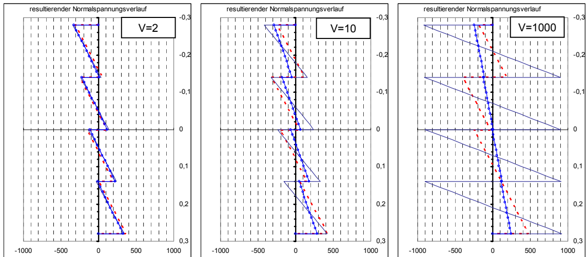
Bild 5.5-26: Normalspannungsverläufe (in Feldmitte) am verdübelten Balken für V=\{2,10,1000\} (bei einer Last von P=1000 kN)
