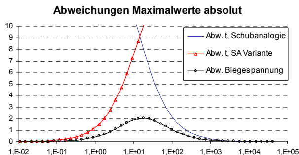
Bild 5.5-5: Absolutwerte für die Abweichungen [%] bezogen auf den maximalen Fugenschub und die maximale Biegespannung in Abhängigkeit von der Fugensteifigkeit [MPa] (Abszisse logarithmisch skaliert)
