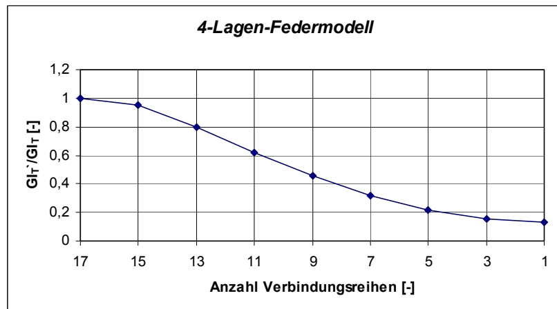
Bild 6.4-4: Vierteiliger Verbundquerschnitt: Verhältnis von effektiver Torsionssteifigkeit GI_T' zur Torsionssteifigkeit GI_T bei starrem Verbund in Abhängigkeit von der Anzahl der Verbindungsreihen (Reduzierung von aussen zur Querschnittsmitte).
