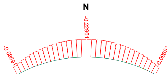
Bild 7.2-24: Querschnitt in Schalenmitte, Normalkraft [\text{kN/Roststab}] bei einer Last von p=3,81 \text{ kN/m}^2 .
