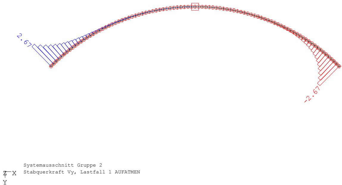
Bild 7.1-4: Querkraftverlauf [kN] am ideellen System, Lastfall „Aufatmen“; Gruppe 1 \equiv Ebene A, Gruppe 2 \equiv Ebene B
