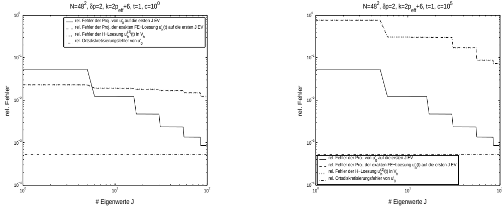
Abbildung 5.2: Relativer algebraischer Fehler der Projektion des Anfangswerts \dot{\mathbf{u}}_0 und der Projektion der exakten FE-Lösung \dot{\mathbf{u}}_h(t) auf \langle \mathbf{v}_1, \dots, \mathbf{v}_J \rangle sowie relativer algebraischer Fehler der \mathcal{H} -Lösung \dot{\mathbf{u}}_h^{(J)}(t) = \sum_{j=1}^J \rho_j^{(\dot{\mathbf{u}}_h(t))} \mathbf{v}_j in V_h und relativer Diskretisierungsfehler im Ort von \dot{\mathbf{u}}_0 zum Zeitpunkt t = 1 in \|\cdot\|_{L^2} für c = 10^0 (links) sowie c = 10^5 (rechts) zu den Anfangsdaten u_0(x_1, x_2) = x_1(x_1 - 1)x_2(x_2 - 1) und \dot{u}_0(x_1, x_2) = 5x_1(x_1 - 1)x_2(x_2 - 1) und der Inhomogenität f \equiv 0 .
