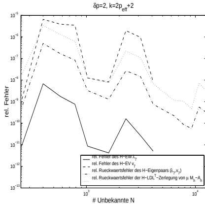
Abbildung 4.7: Relativer Fehler der \mathcal{H} -EW \lambda_7 (links) und \lambda_8 (rechts) und der zugehoerigen \mathcal{H} -EV \mathbf{v}_7 (links) und \mathbf{v}_8 (rechts) sowie relativer R ckw rtsfehler der \mathcal{H} -Eigenpaare (\lambda_7, \mathbf{v}_7) (links) und (\lambda_8, \mathbf{v}_8) (rechts) in \|\cdot\|_2 und relativer R ckw rtsfehler der \mathcal{H} - LDL^T -Zerlegung von \mu M_h - A_h in \|\cdot\|_F f r \delta p = 2 und Rang k = 2p_{eff} + 2 .
