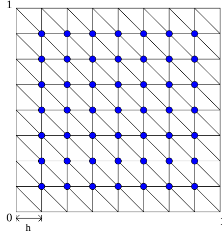
Abbildung 3.2: Regelmäßig trianguliertes Einheitsquadrat mit h = \frac{1}{n+1}
