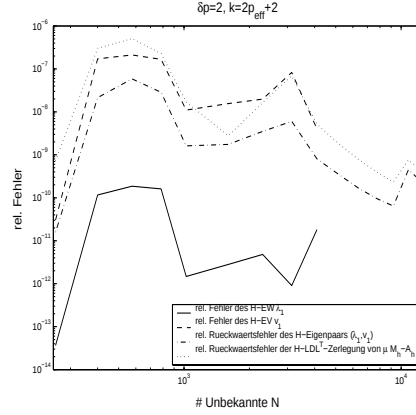
Abbildung 4.6: Relativer Fehler des \mathcal{H} -EW \lambda_1 und des zugehoerigen \mathcal{H} -EV \mathbf{v}_1 sowie relativer R ckw rtsfehler des \mathcal{H} -Eigenpaars (\lambda_1, \mathbf{v}_1) in \|\cdot\|_2 und relativer R ckw rtsfehler der \mathcal{H} - LDL^T -Zerlegung von \mu M_h - A_h in \|\cdot\|_F f r \delta p = 2 und Rang k = 2p_{eff} + 2 .
