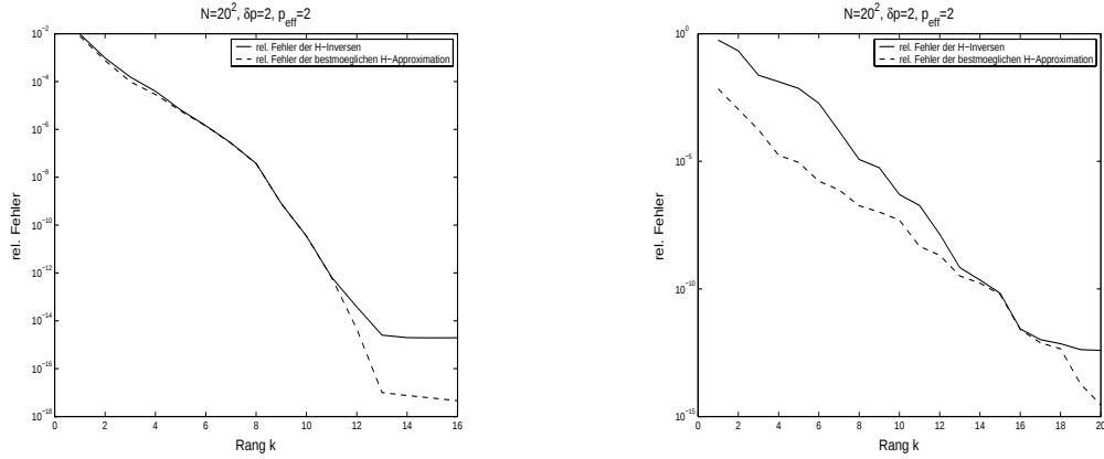
Abbildung 3.11: Relativer Fehler der \mathcal{H} -Inversen von A_h (links) und von A_h^2 (rechts) sowie der bestmöglichen \mathcal{H} -Approximation an die exakte Inverse von A_h (links) und von A_h^2 (rechts) in \|\cdot\|_F .
